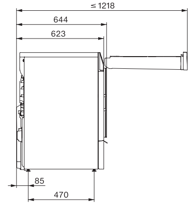
T2 mit Glastür, 17 Grad Blende, mit QuickPowerDry, Maße in mm
